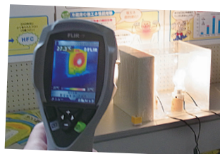
サーモカメラを活用した 断熱性能比較
